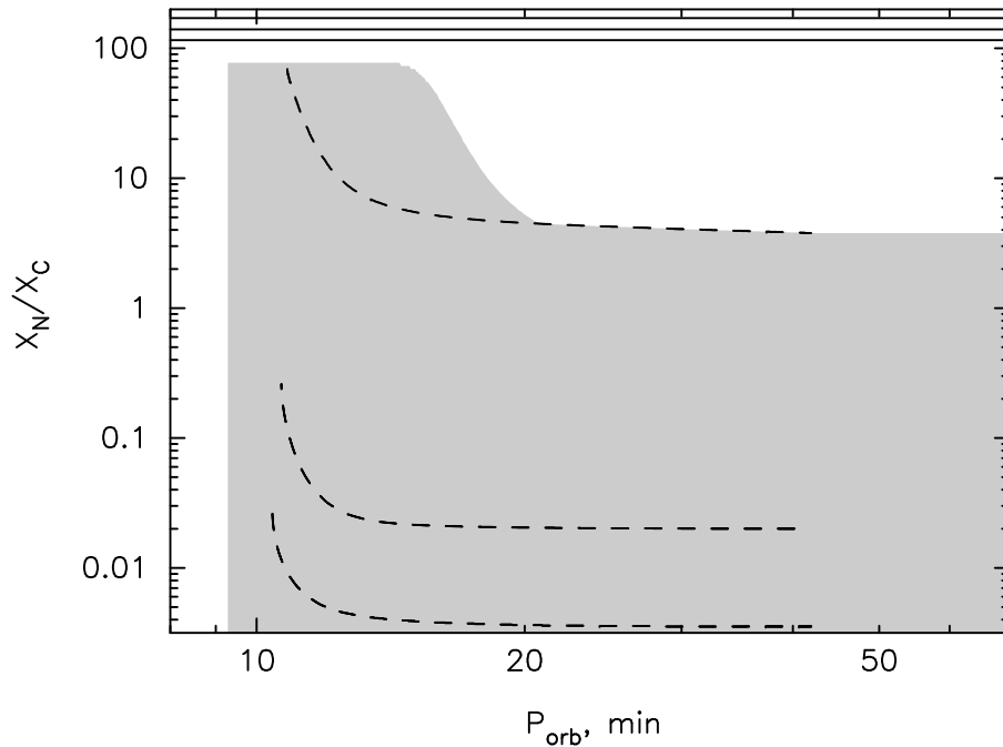
Рис. 4: Отношение содержаний N и C в аккреционных дисках звезд AM CVn при различных значениях P_{\text{orb}} . Прямые линии соответствуют донорам-карликам с массами предшественников 1, 1.5, 2 M_{\odot} (сверху вниз). Если донор — гелиевая звезда, X_N/X_C может иметь значения, соответствующие затененной области, вплоть до 0. Штриховые линии — примеры эволюции X_N/X_C .
