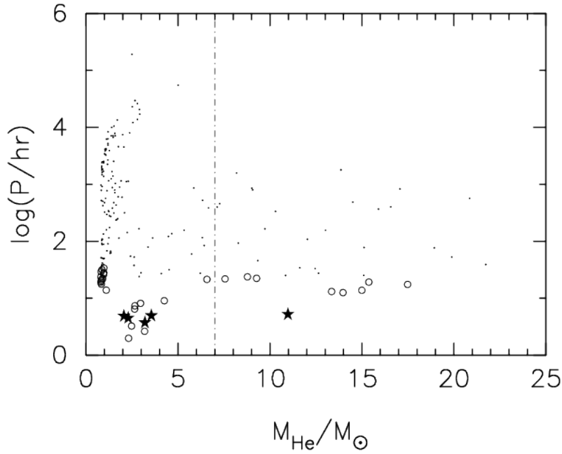
Рис. 6: Соотношение между массами гелиевых звезд M_{\text{He}} и орбитальными периодами систем из гелиевых звезд и черных дыр. Кружками отмечены системы с дисками. Звездочки – системы с P_{\text{orb}} = 4.8 \pm 1.2 , т. е. близкие к Cyg X-3. Вертикальная линия — нижний предел масс звезд WR.
