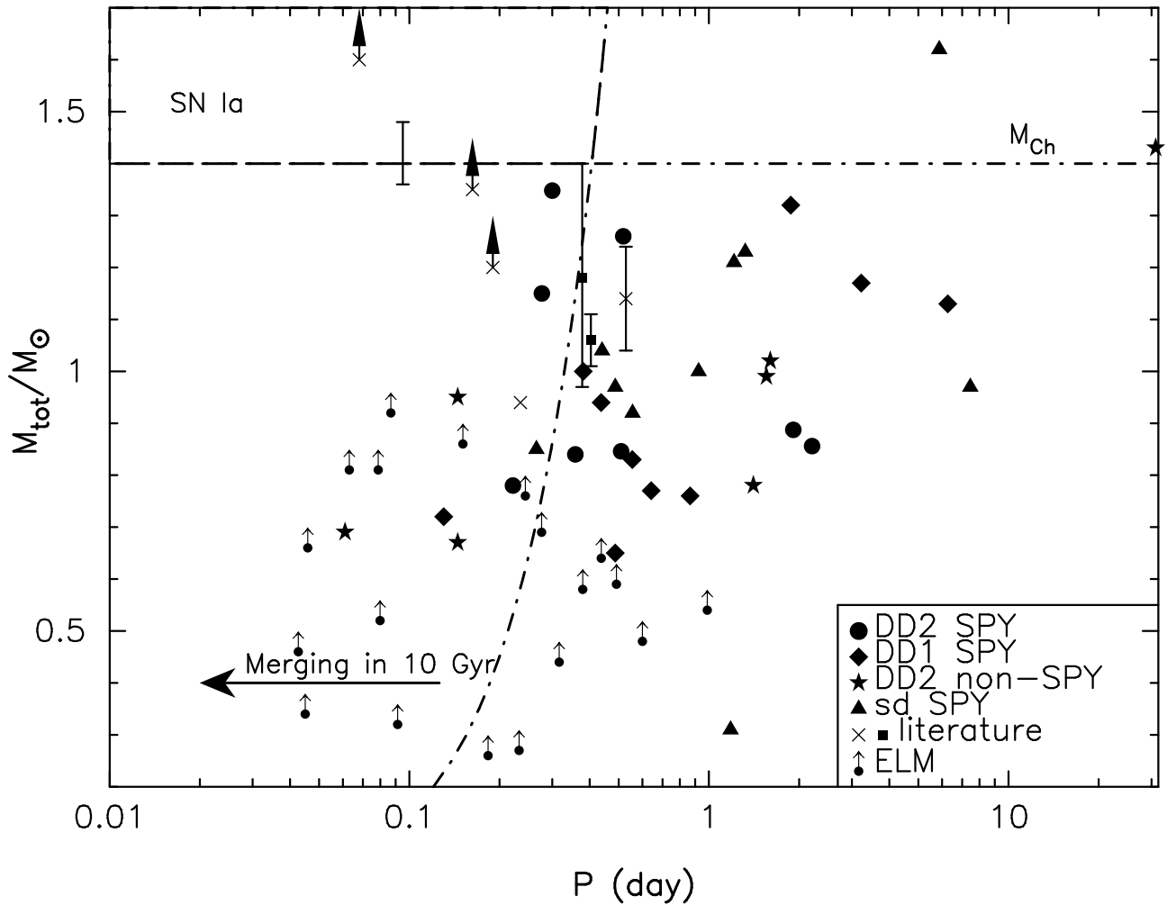
Рис. 1: Полные массы известных двойных БК и горячих субкарликов со спутниками–БК. DD2 — системы с двумя видимыми спектрами. Для систем с одним видимым спектром (DD1) показаны нижние пределы M_{tot} . Кружки со стрелками — нижние пределы M_{tot} для БК экстремально малых масс, отождествленных в SDSS (ELM). Отмечены M_{Ch} и предел периодов, при котором слияние происходит за время, меньшее 10^{10} лет. Возможные предшественники СН Ia (SN Ia) расположены в верхнем левом углу рисунка. Выделены системы, найденные в проекте SPY.
