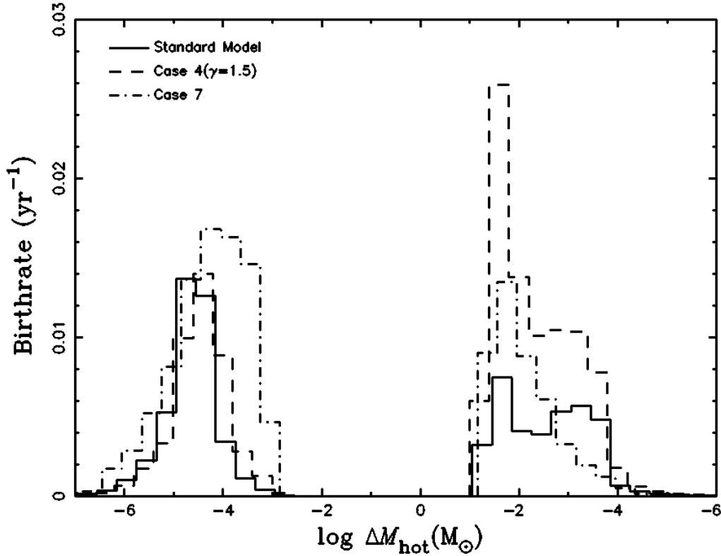
Рис. 7: Распределение симбиотических звезд по эффективности аккреции (справа от 0.0) или эрозии (слева от 0.0). Модели соответствуют различным значениям параметра общих оболочек \alpha_{ce} и \gamma , скорости звездного ветра, эффективности аккумуляции вещества.
