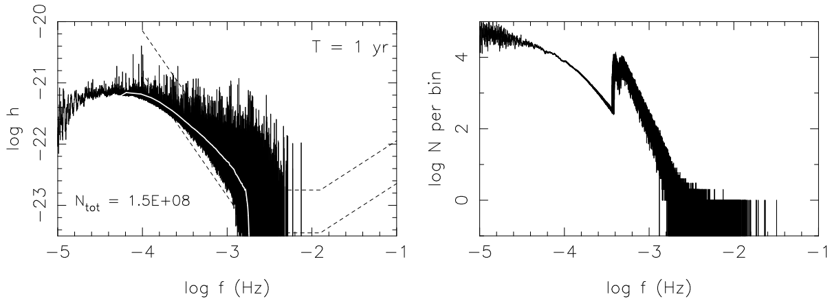
Рис. 5: Слева — гравитационно-волновой фон, создаваемый БК, справа — численность систем в единичных полосах пропускания детектора. Белая линия — усредненный фон, штриховые линии — пределы чувствительности детектора для периодов наблюдений 1 год и 5 лет.
