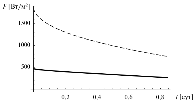
Рис. 13б. Потoki скрытого (сплошная линия) и явного (пунктирная линия) тепла [Вт/м 2 ] в полярной области
